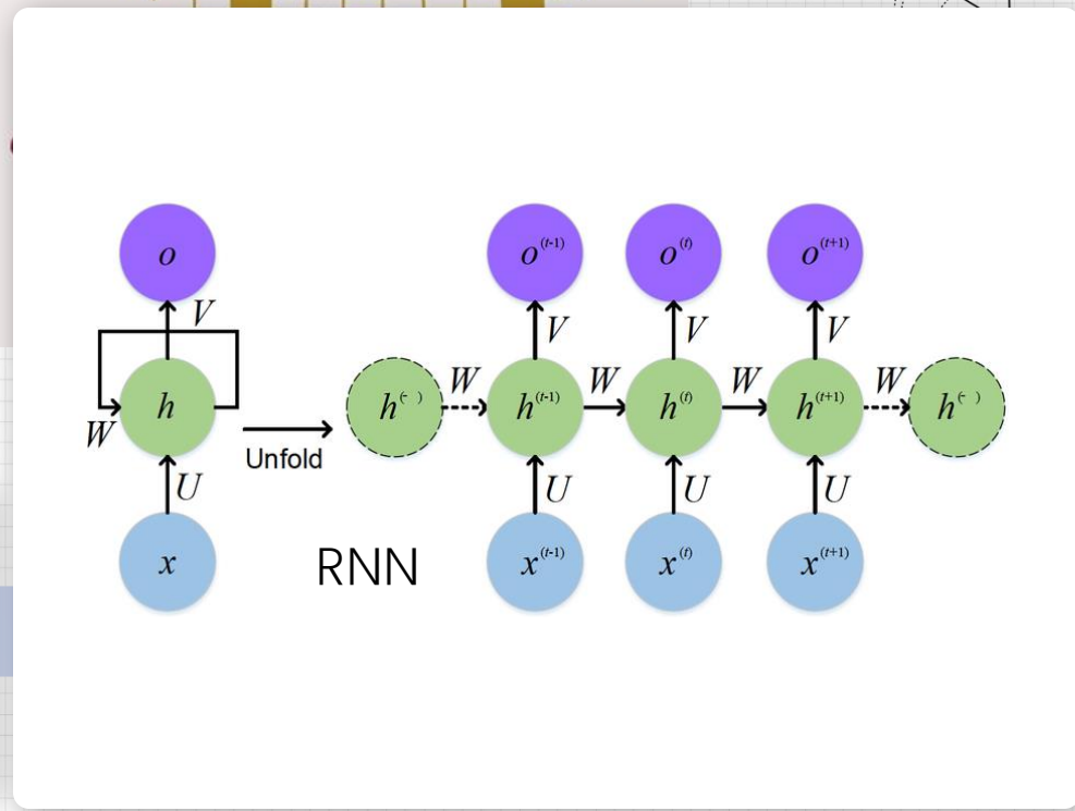
神经网络时代 (RNN)
